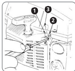
1. Igła L 2. Igła H 3. Śruba (T) regulacji biegu jałowego
